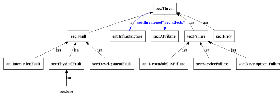
Fig. 2. Sub-tree 'sec:Threat'
